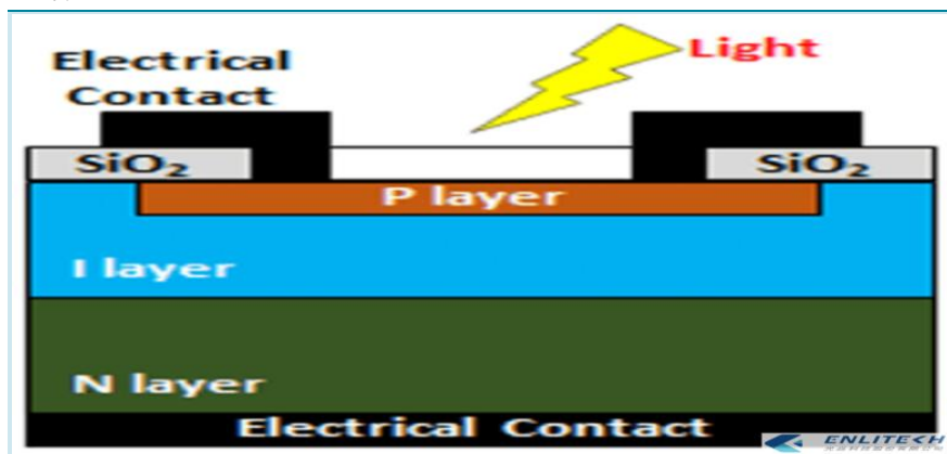
圖表 6:PD 結構圖
