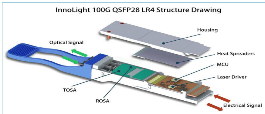
圖表 7:光收發模組結構圖
